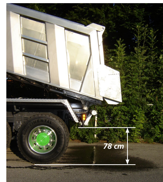
Schüttblech für Einbaumaschine
